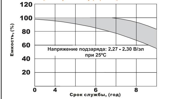
Срок службы в буферном режиме
