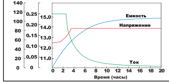
Заряд постоянным напряжением (0,3СА, 25°C)
