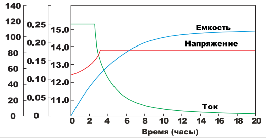
Заряд постоянным напряжением (0.25СA, 25°C)
